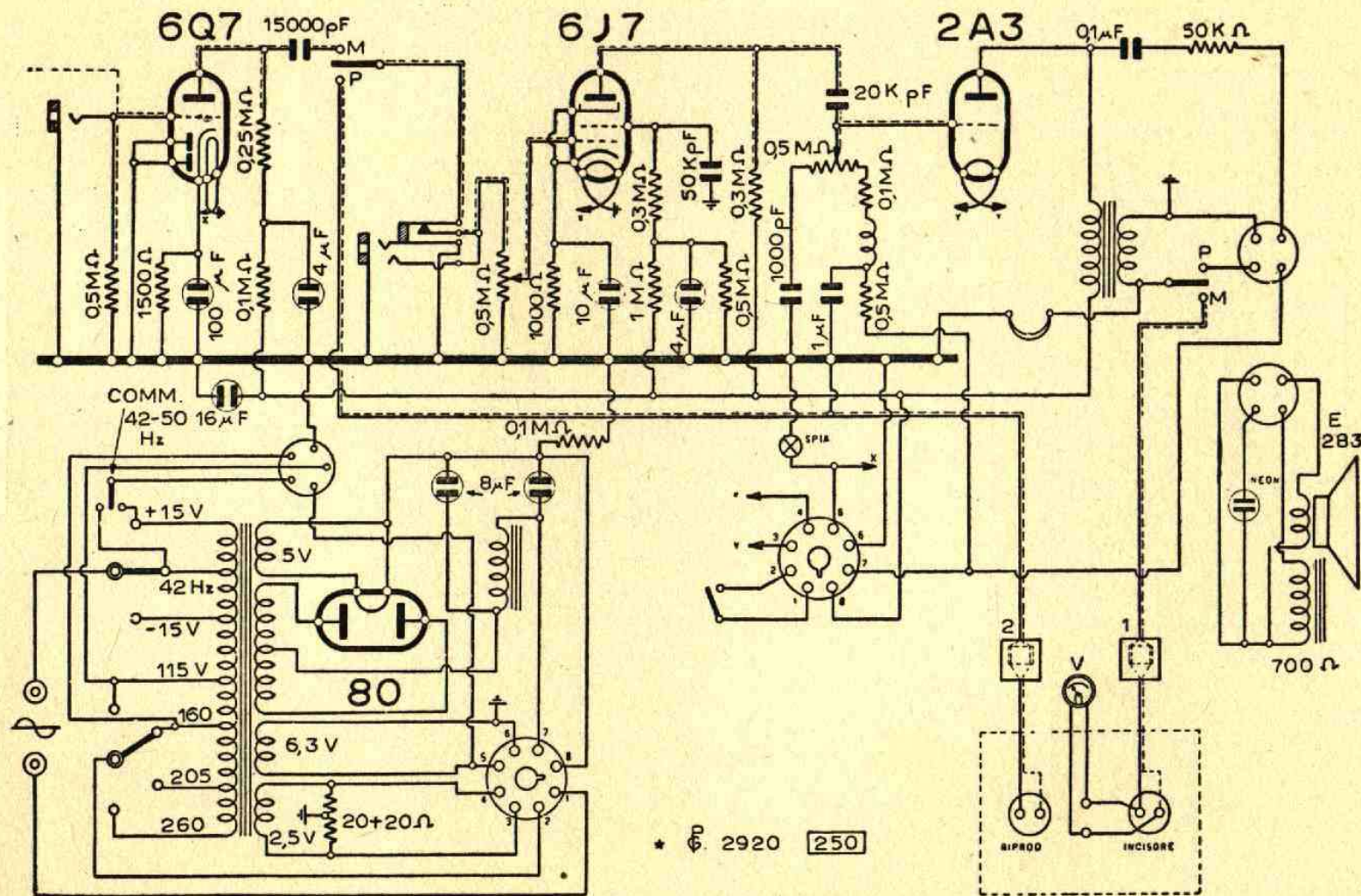
Lo schema elettrico del Fonoincisore mod. 44.
